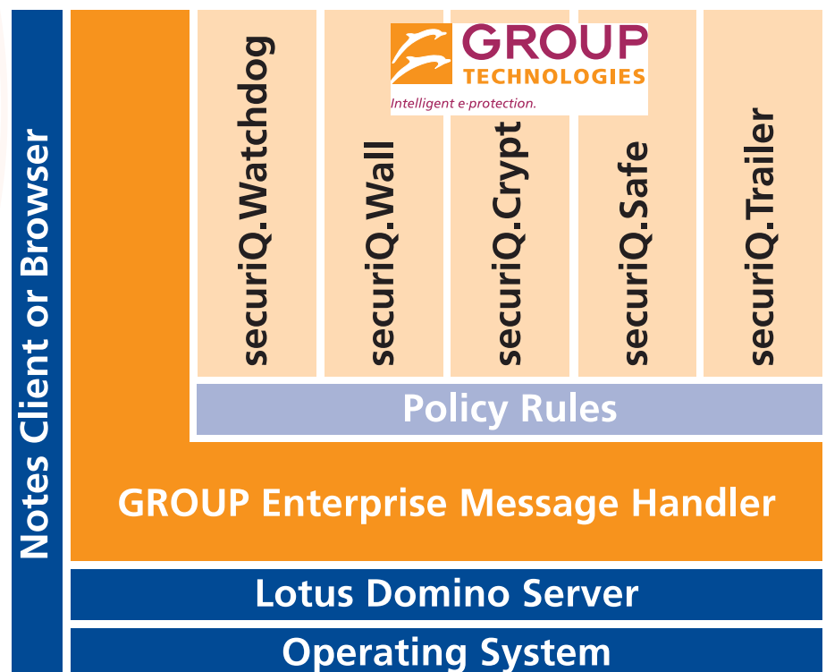
Architektur der securiQ. Suite
